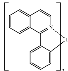
Ir(piq) 3
