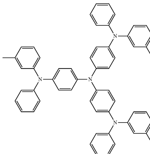
m-MTDATA
