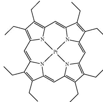
PtOEP
